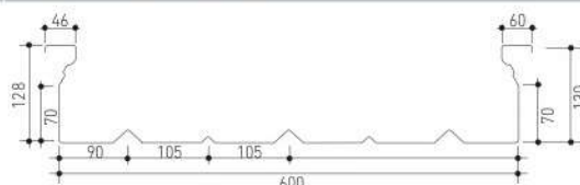
SECCIÓN PERFIL
