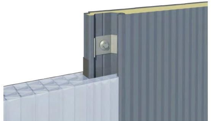
DETALLE ENTREGA ENTRE PLACAS DE POLICARBONATO - PANEL METÁLICO
