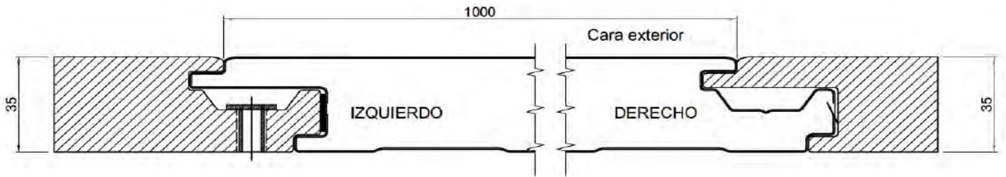
DETALLE ENTREGA POLICARBONATO - PANEL FACHADA - FIJACIÓN OCULTA
