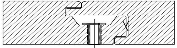
DETALLE ENTREGA ENTRE PLACAS DE POLICARBONATO - CASQUILLO FIJACIÓN PANEL
