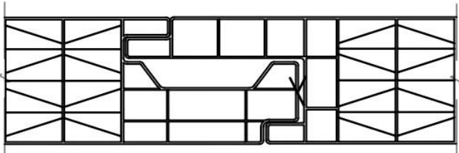
DETALLE ENTREGA ENTRE PLACAS DE POLICARBONATO - CASQUILLO FIJACIÓN PANEL
