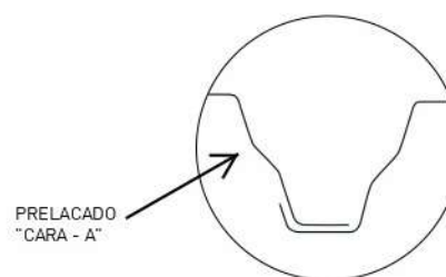
DETALLE SOLAPE
