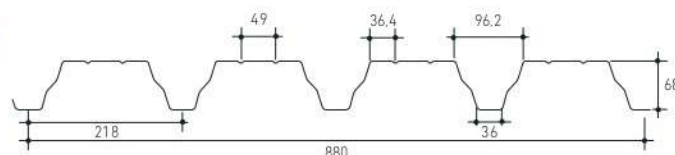
SECCIÓN PERFIL
