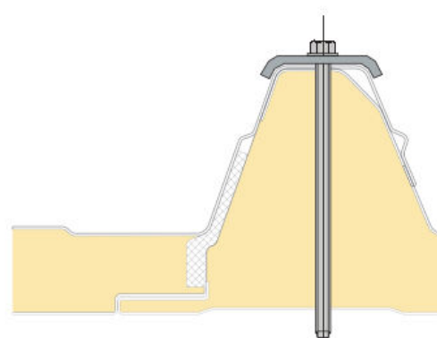
DETALLE SOLAPE LONGITUDINAL
