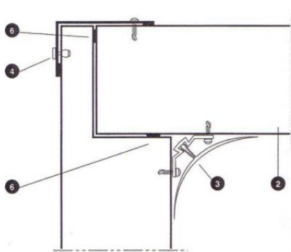
ARRANQUE PANEL CONSERVACIÓN
