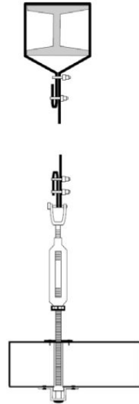
EJEMPLO DE SISTEMA DE CUELGUE A TECHO
