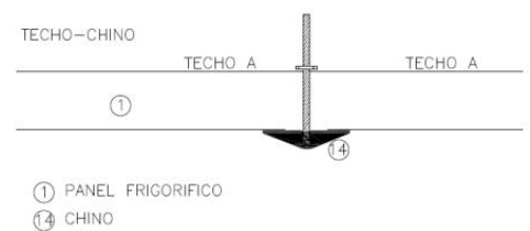
SUSPENSIÓN TECHO POR CHINO
