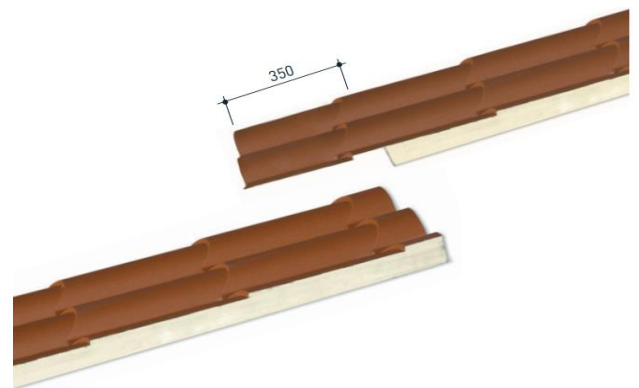
DETALLE SOLAPE TRANSVERSAL
