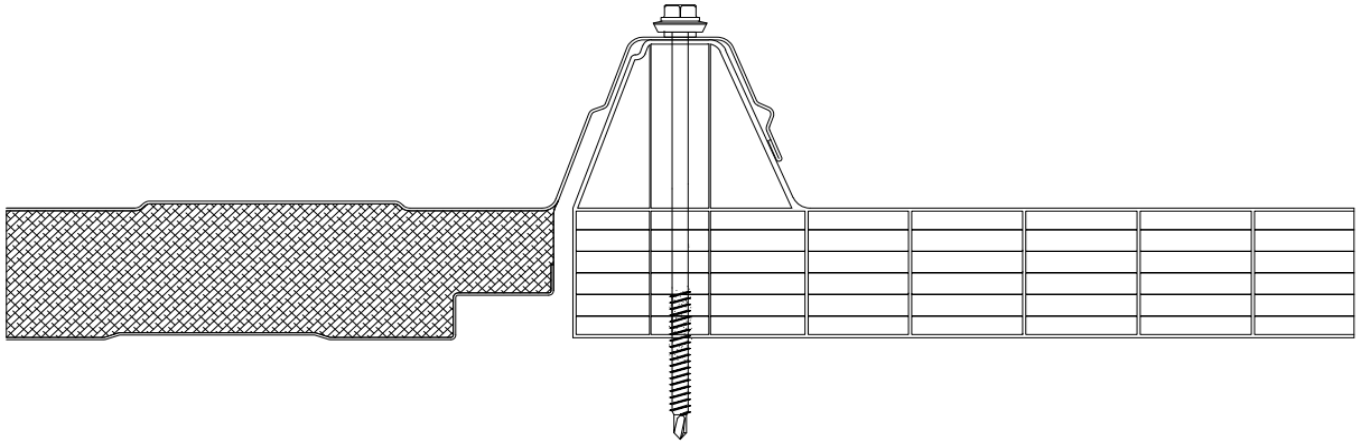
DETALLE ENTREGA POLICARBONATO - PANEL DE CUBIERTA 3GR/5GR ST
