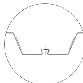
DETALLE SOLAPE
