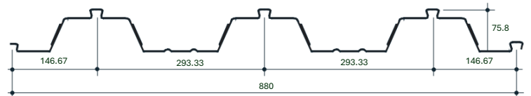
SECCIÓN PERFIL
